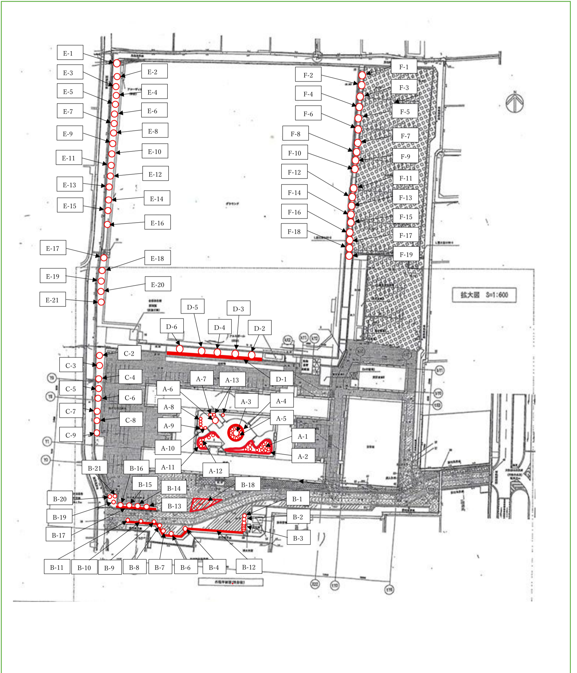
令和7年度郡山総合庁舎植栽配置図
