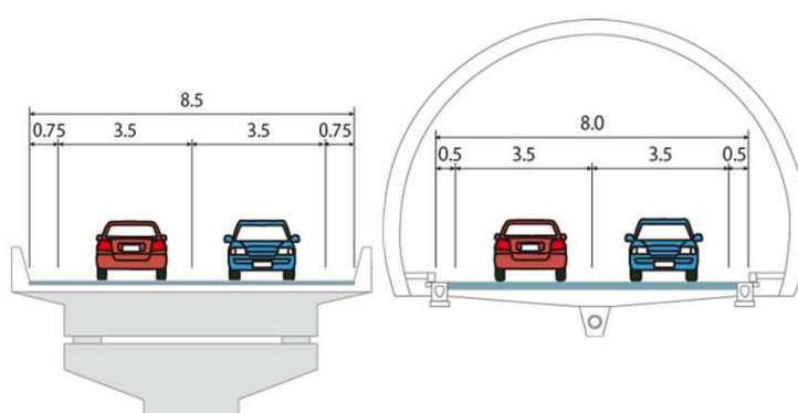
【橋梁部】
