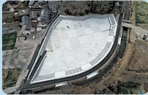
川合調整池（河合町） 貯留量 11,000 m 3
