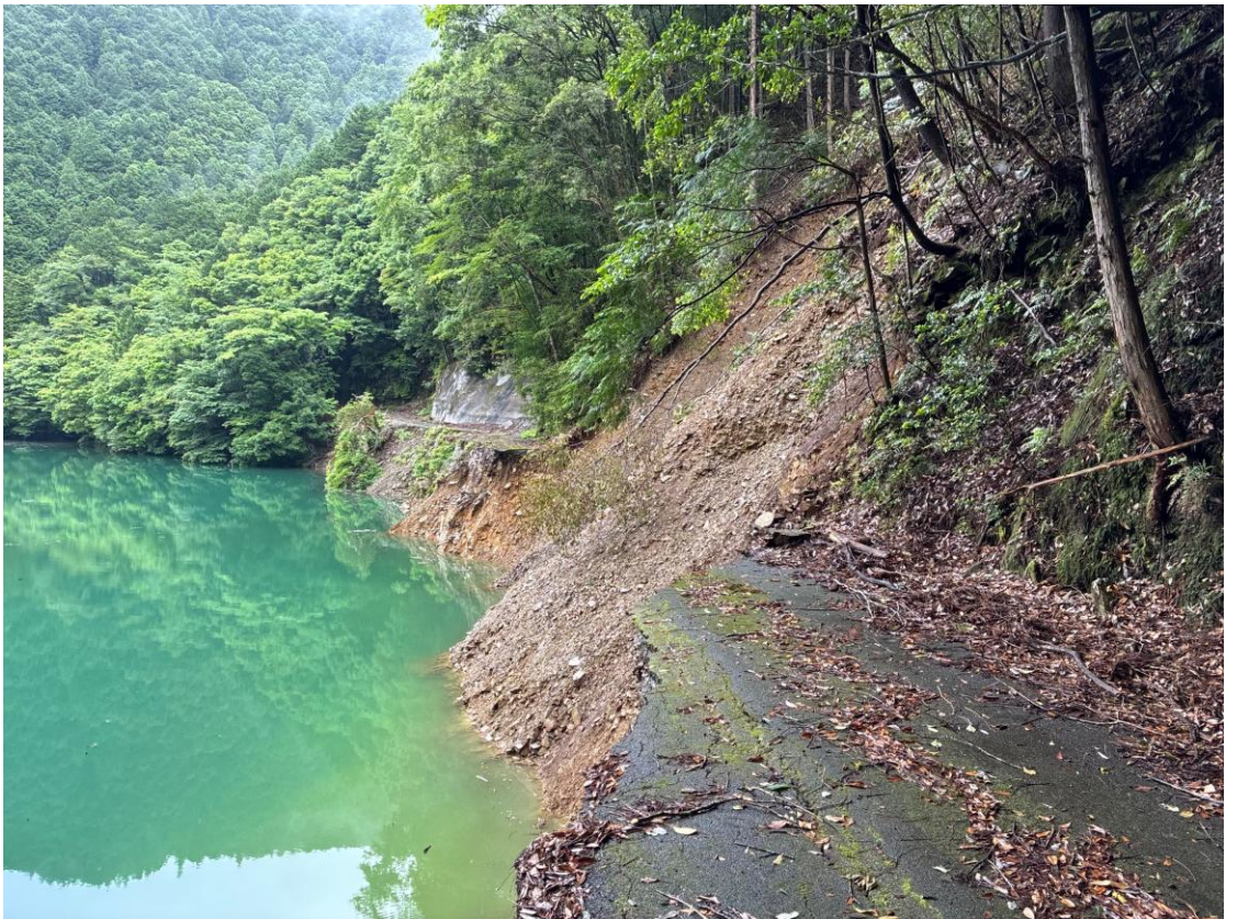
法面崩落
