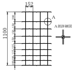
SGクロスフェンス 943-6SSa
