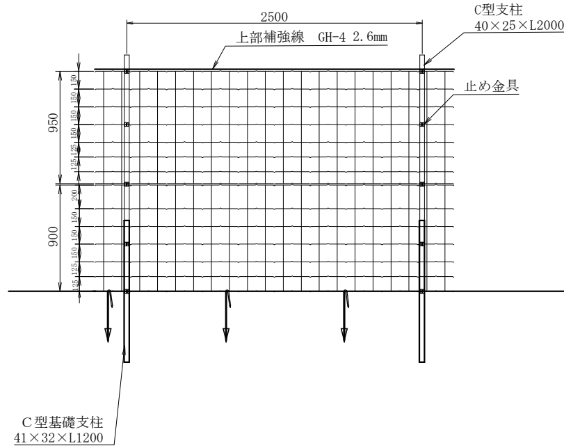
SGクロスフェンス 943-6SSa
