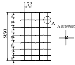
SGクロスフェンス 838-6SSa
