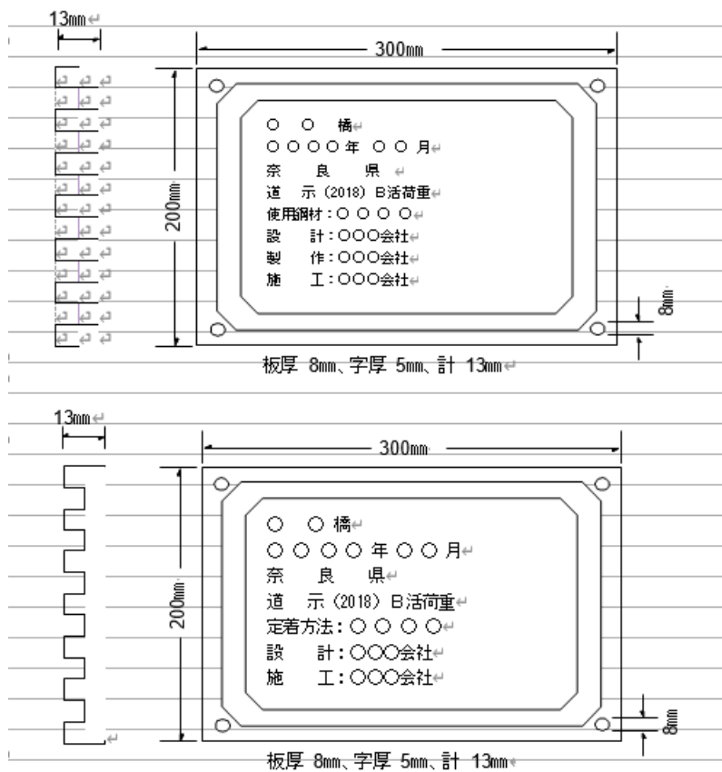
図3-2-2 銘板の寸法及び記載事項
