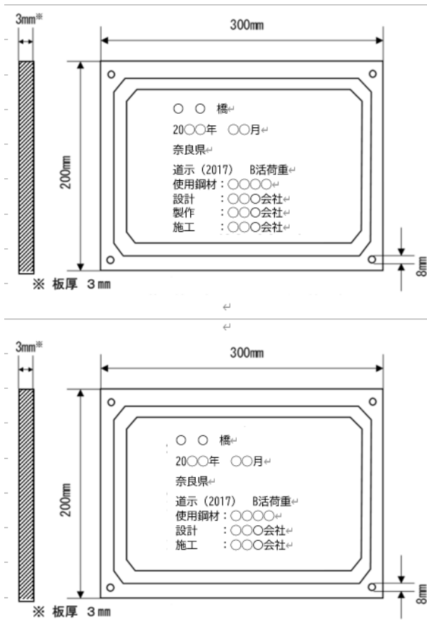
図3-2-2 銘板の寸法及び記載事項
