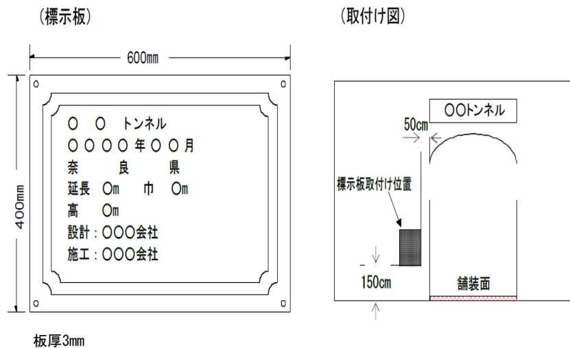
図10-6-2 標示板の設置イメージ図
