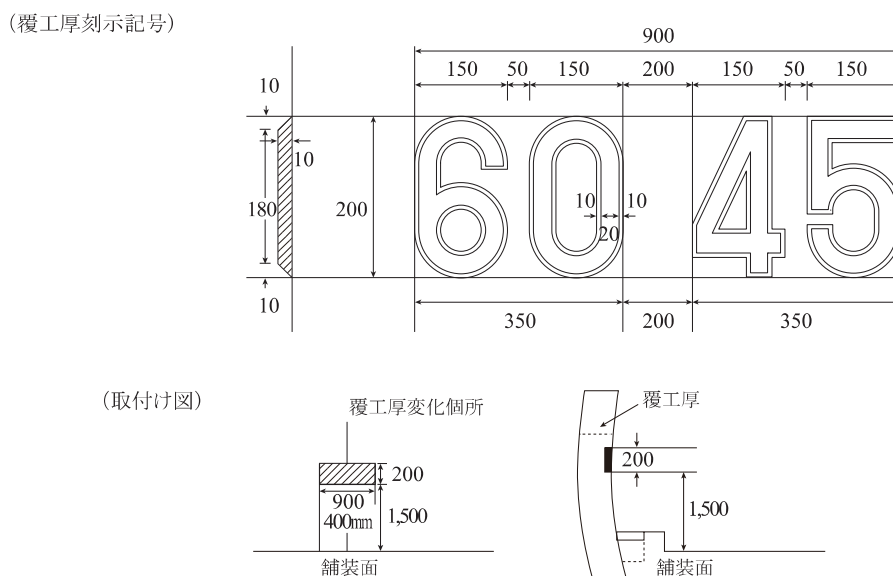
図10-6-1 覆工厚変化箇所の特示標準図
