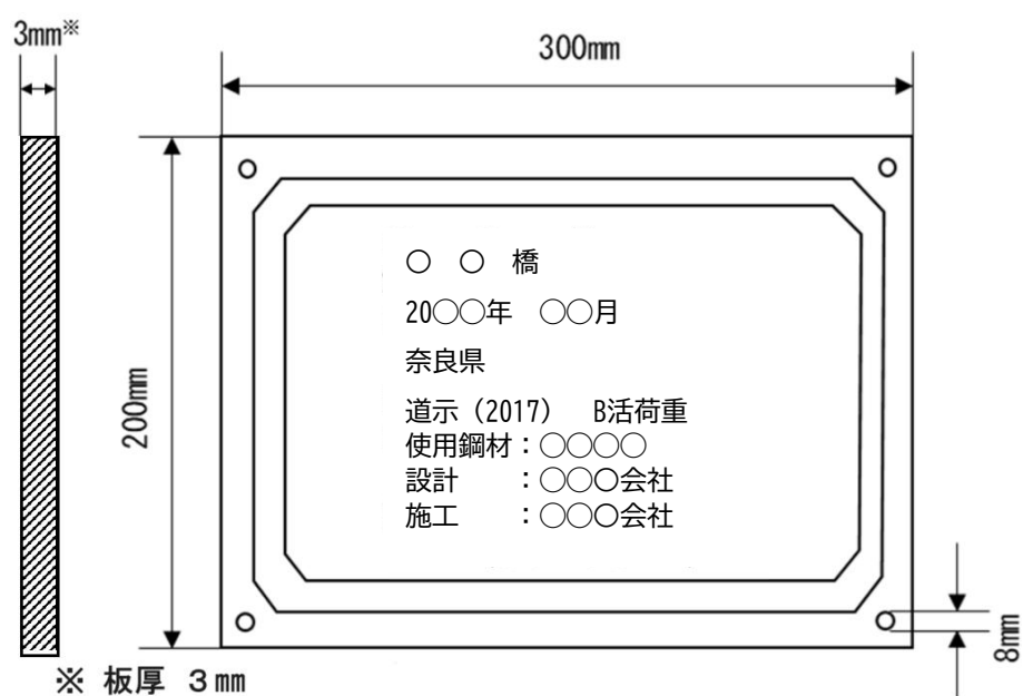
図3-2-2 銘板の寸法及び記載事項
