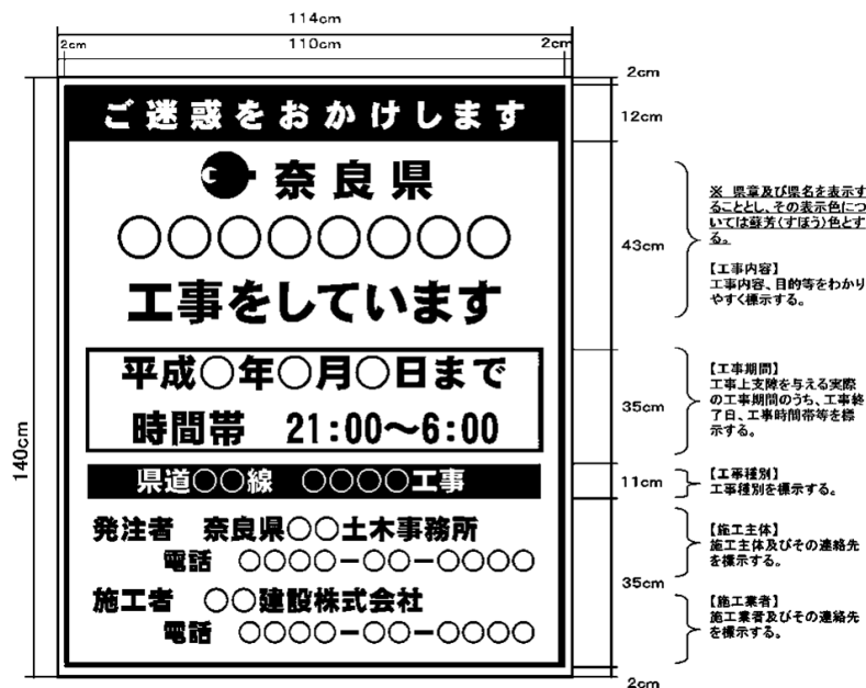
図1-1-2 標示板の例
