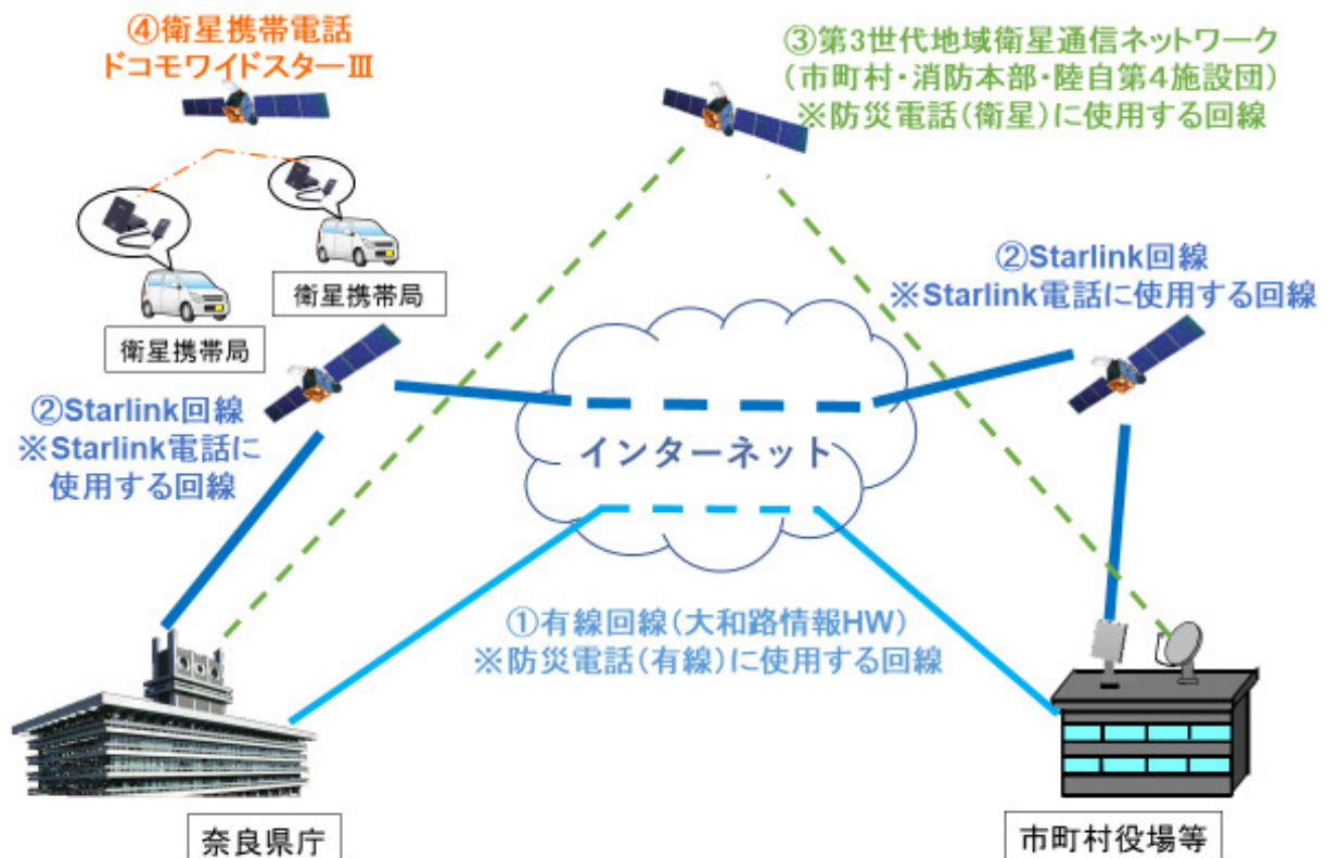
奈良県防災行政通信ネットワーク（イメージ図）
